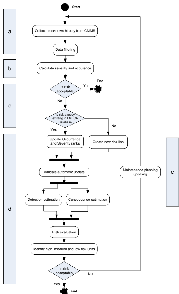
Figure 4 Nouvelle approche pour la RBM : RBMd
